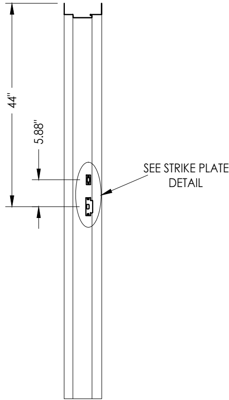
STRIKE JAMB
