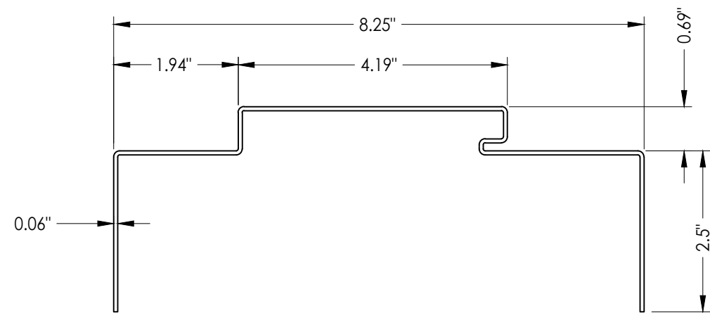
1 FRAME 16 GA.
